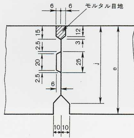
接合部詳細図
