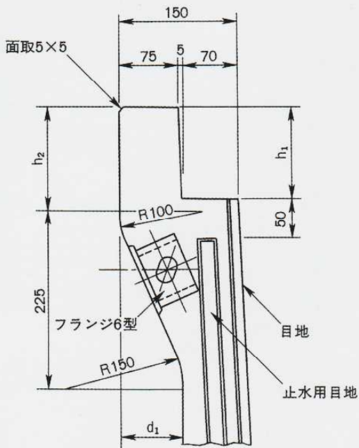
側板の天端部詳細図
