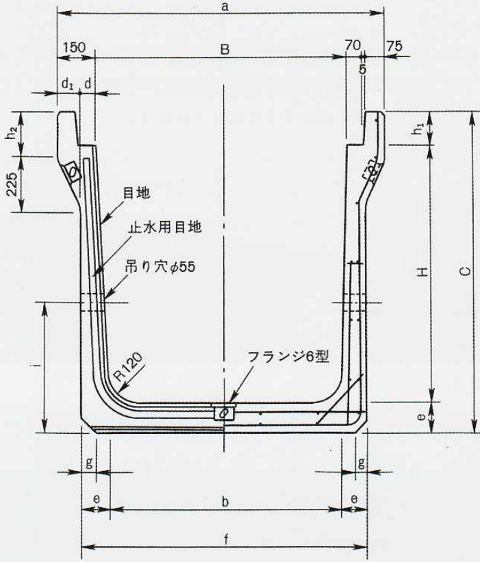
断面図
