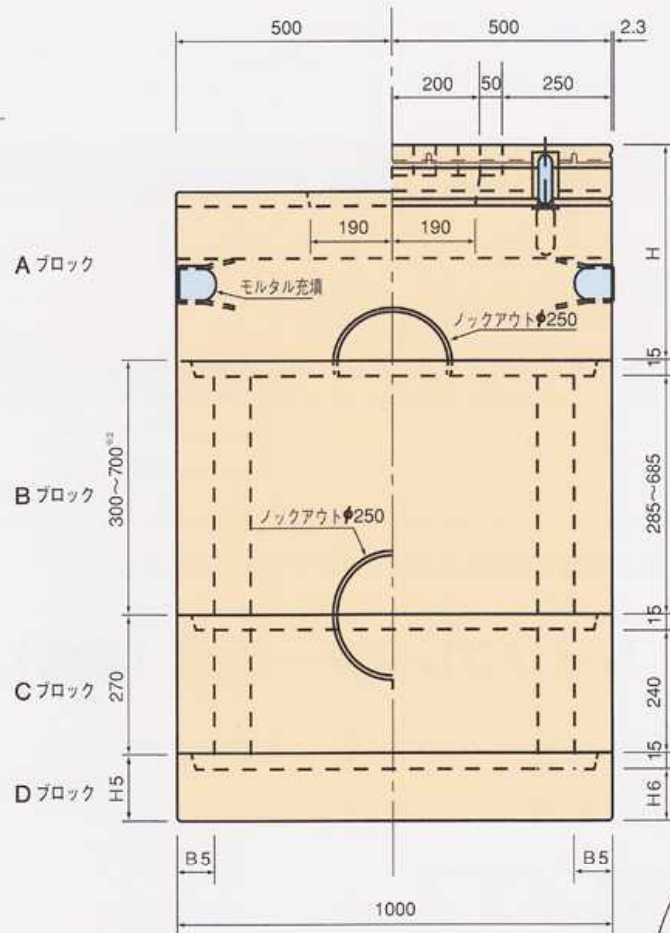
左側側面図
