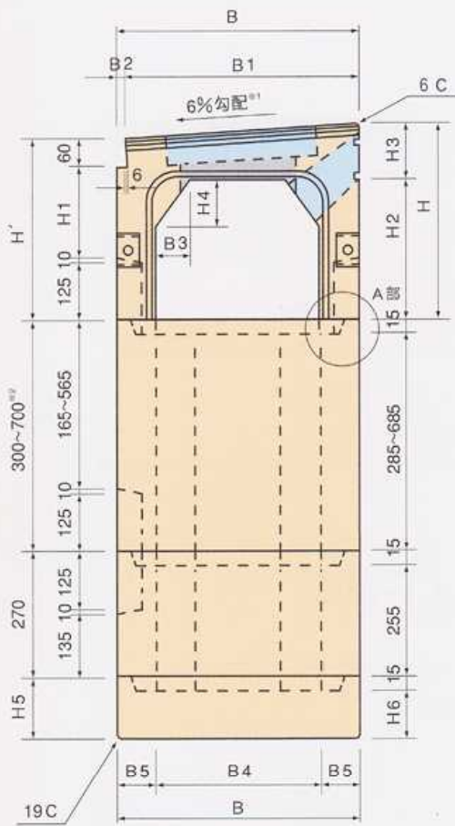
正面図
